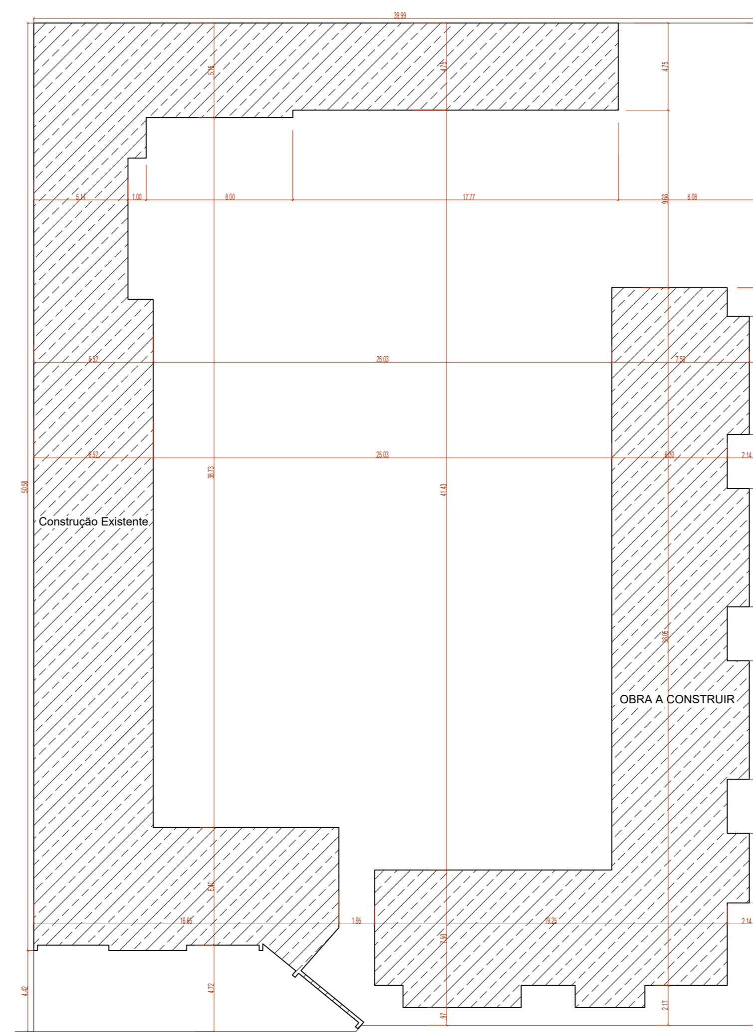
6 Planta de Implantação Esc.: 1/200
