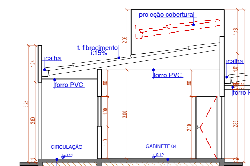
4 Corte AA Esc.: 1/75
