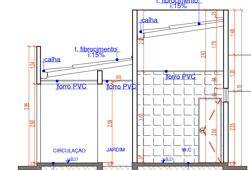
5 Corte BB Esc.: 1/75
